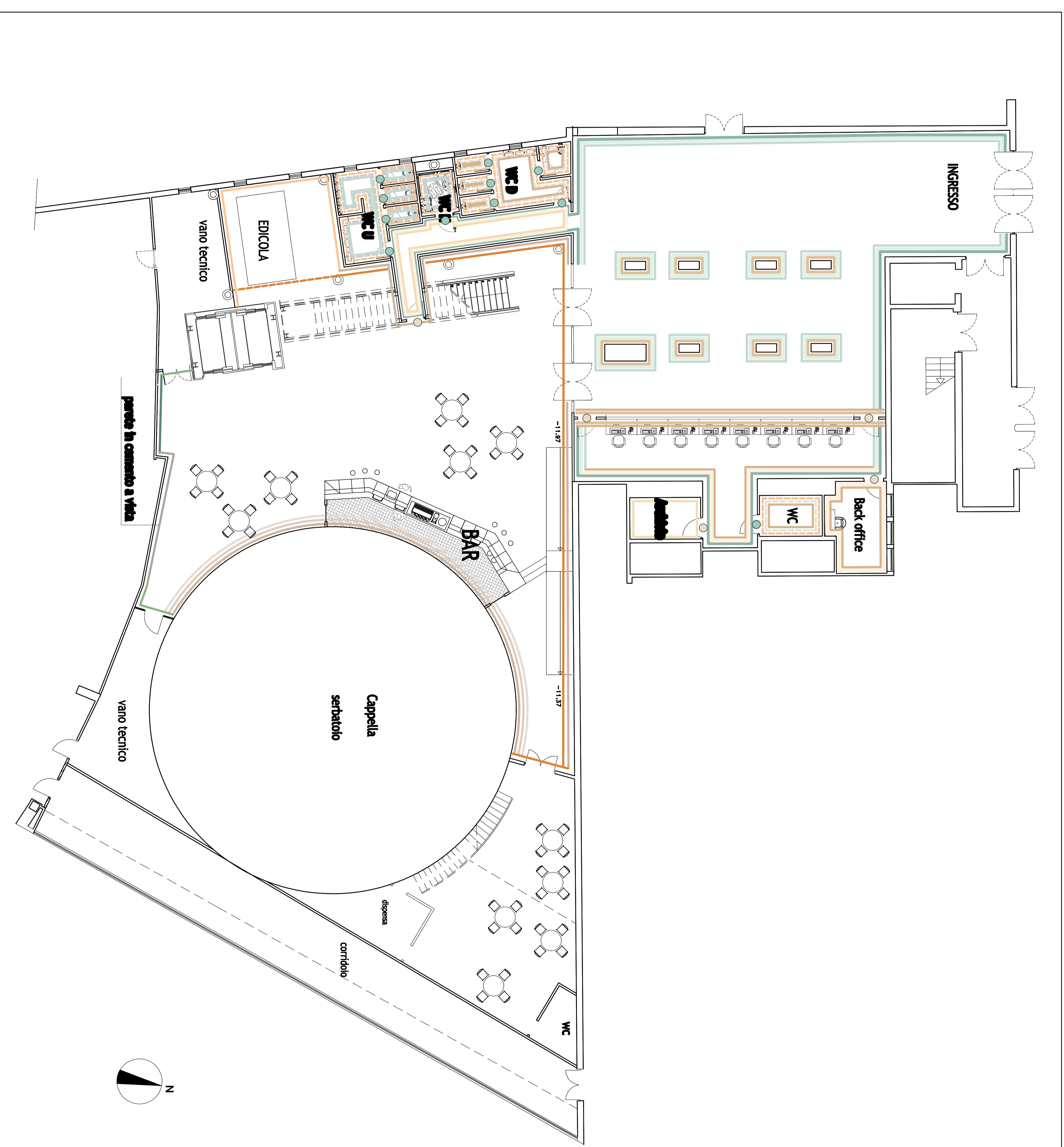
Planta RIVESTIMENTI rapp. 1:100
